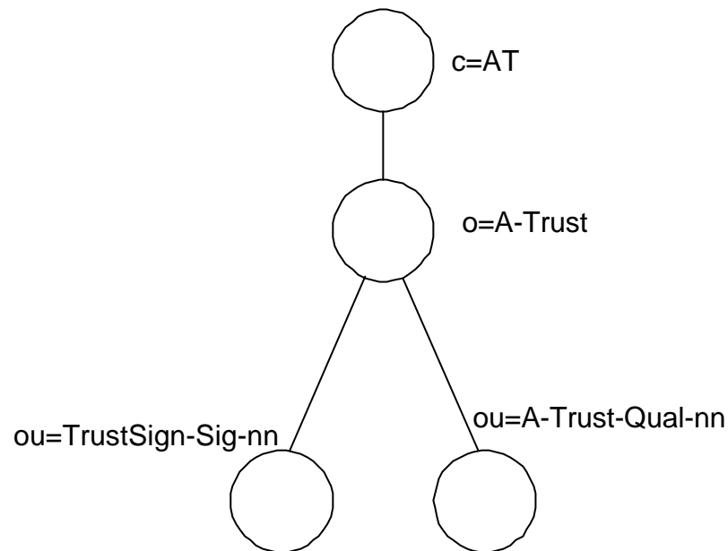
Abbildung 2 Verzeichnisbaum
